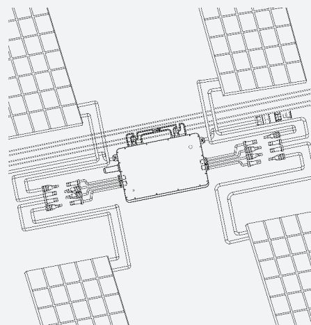
Rys. 1 Pozycja instalacyjna mikroinwertera
