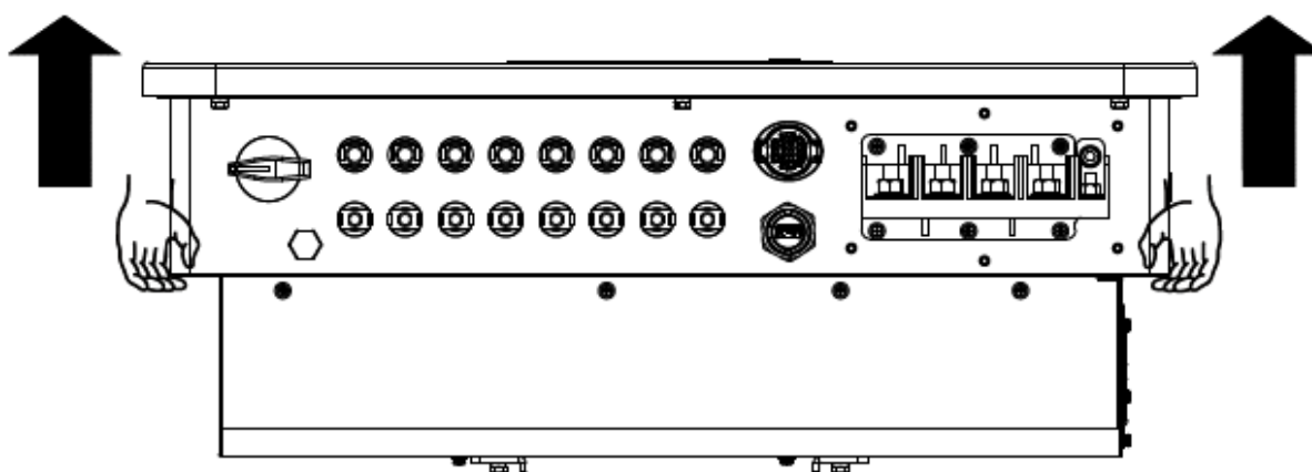
Rysunek 3-5: Wyjmowanie falownika z opakowania (2)
