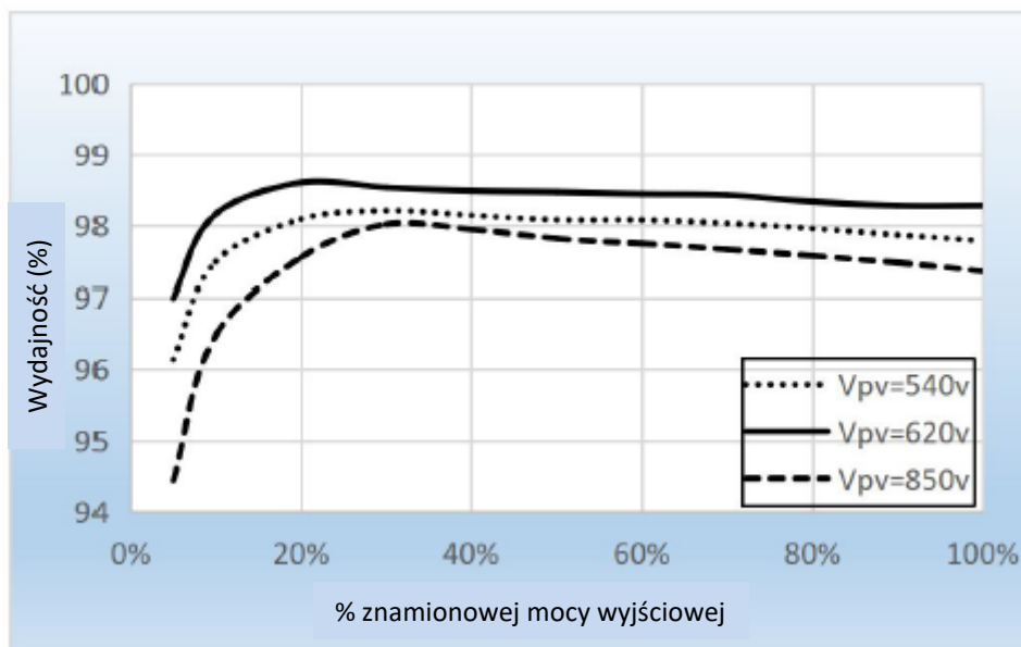
Rysunek 2-9: Krzywa wydajności (na przykładzie 50 kW)
